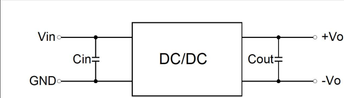
应用电路（图 3）
