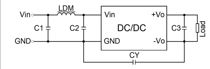
应用电路（图 4）
